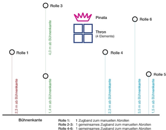
Skizze der Elemente im Grundriss
